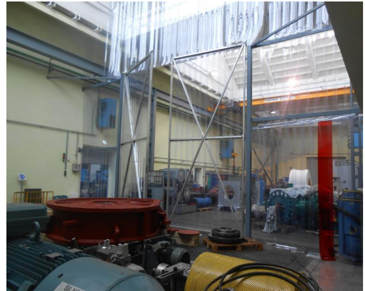
Stacja prób wyposażona w kurtynę dźwiękochłonną z lameli PCV
